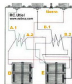
ACOPLADOR Fig.52
